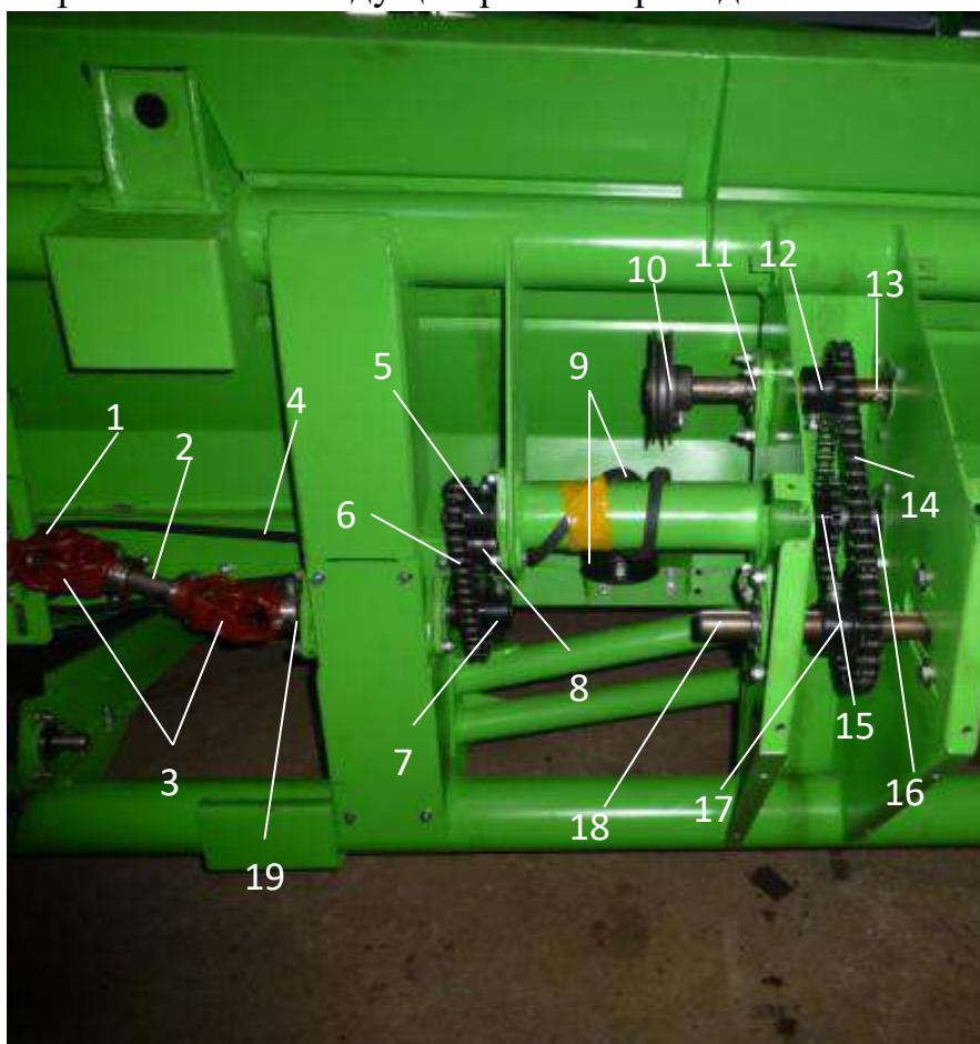
Рис.14 Привод правого транспортёра и битера жатки.
