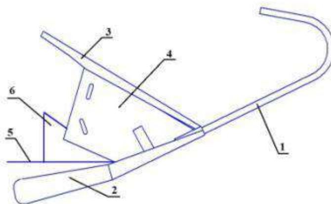
Рис.27 Зерноделитель.
