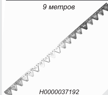
Нож «Шумахер»
